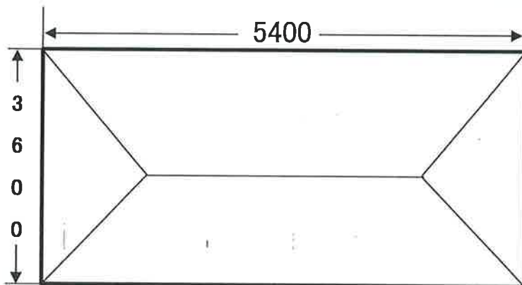
2間×3間/6坪テント(3600×5400)
